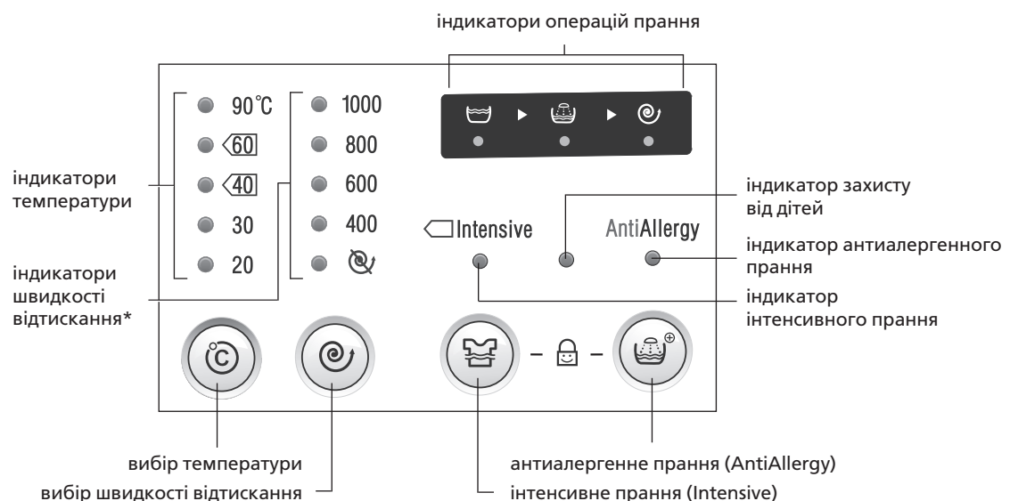
Рисунок 1 – Панель керування
