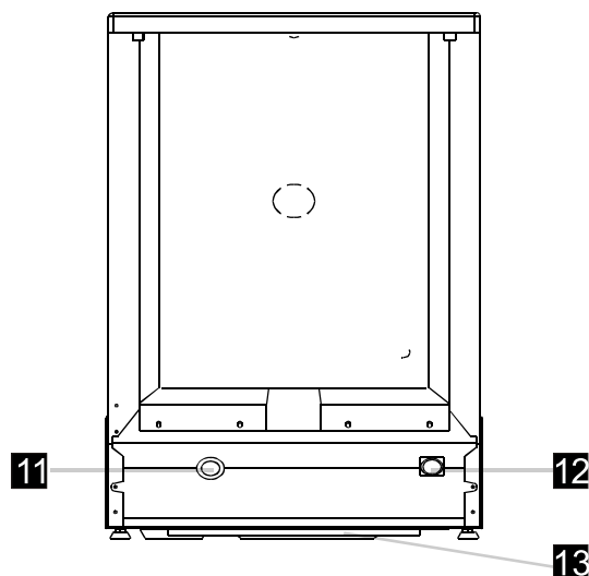
Вид сзади
