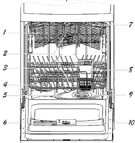
Čelní pohled
