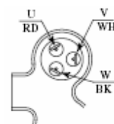
Схема выходов компрессора
