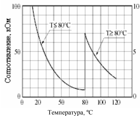
Температурная характеристика сопротивления для термистора транзистора питания (Tho-D)
