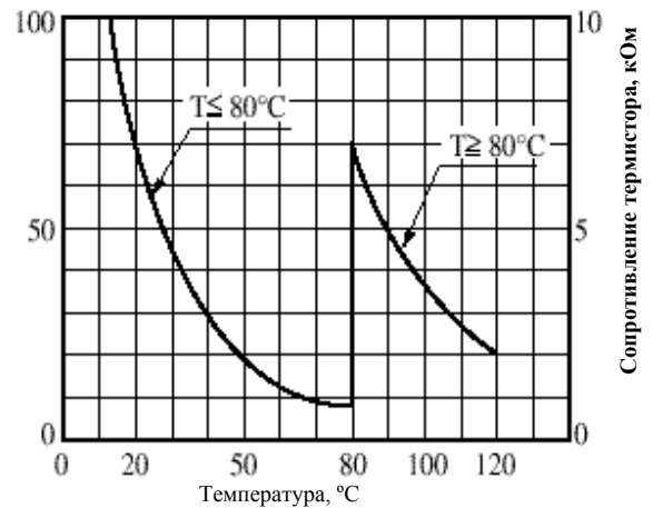
Температурная характеристика сопротивления для термистора спускной трубы (Tho-A)
