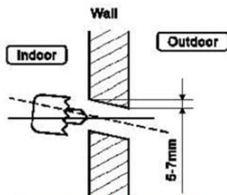
Wall - стена, Indoor - помещение, Outdoor – улица, 5-7 mm – 5-7 мм
