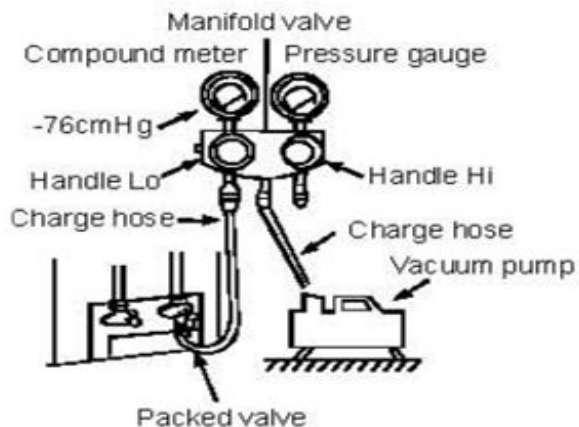
Manifold valve - распределительный клапан, compound meter - индикатор разряжения, pressure gauge - манометр, -76cmHg -76 см рт. ст., handle Lo - маховичок низкого давления, handle Hi - маховичок высокого давления, charge hose - нагнетательный шланг, vacuum pump - вакуумный насос, packed valve - герметизирующий клапан
