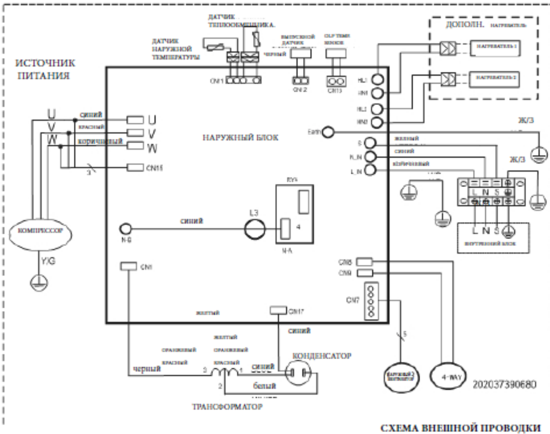
СХЕМА ВНЕШНЕЙ ПРОВОДКИ
