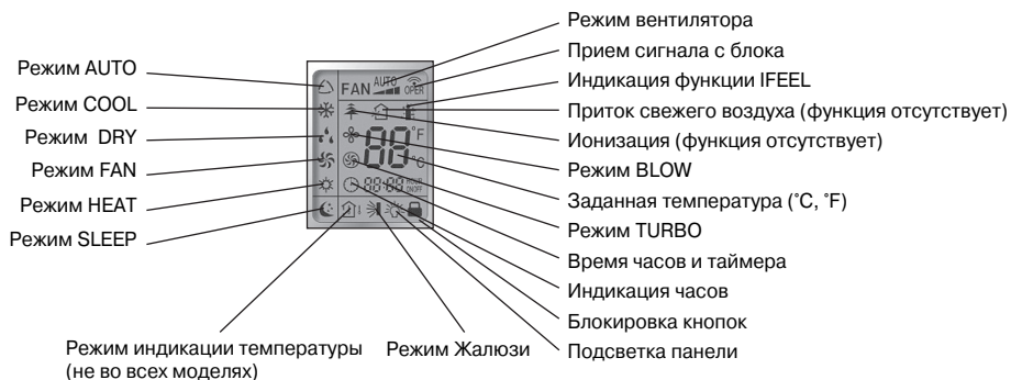
Рис. 5.1.1 Индикация пульта
