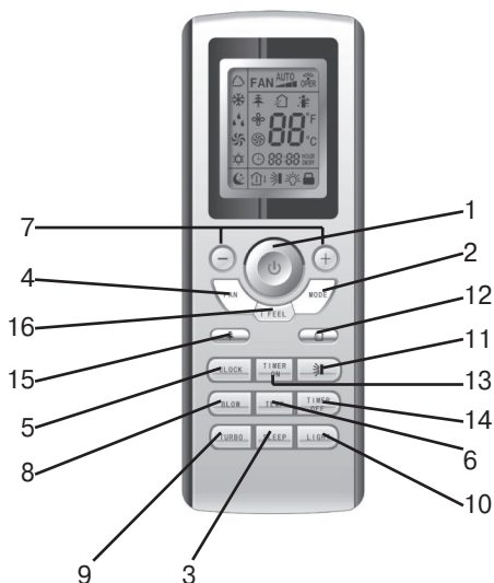
Рис. 5.9 Пульт управления
